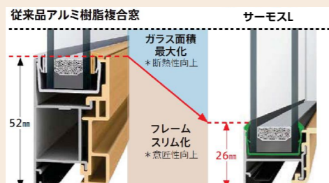
※画像は引違い窓の縦枠です。
